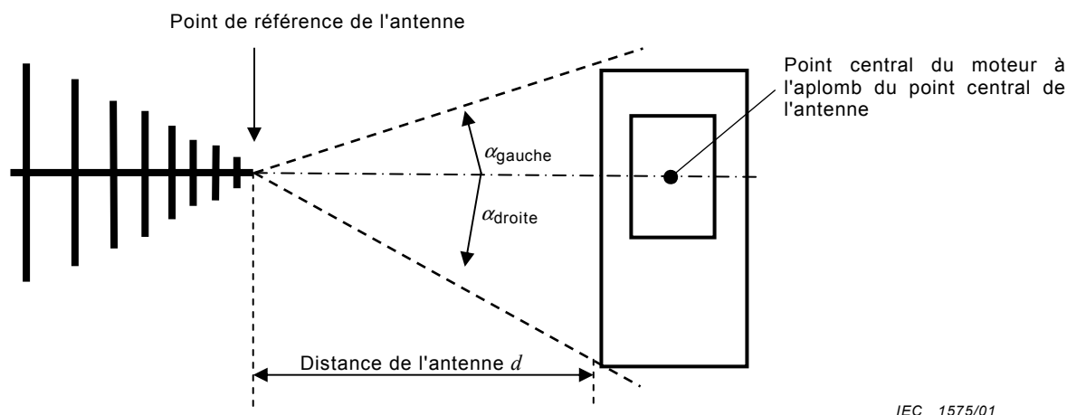
Figure H.1 – Détermination de l'angle maximal à couvrir par l'antenne
