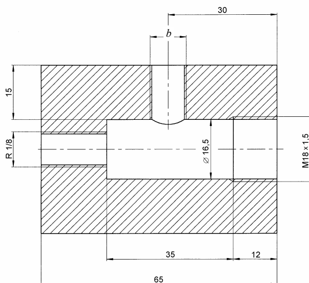
Figure F.3a – Vue générale
