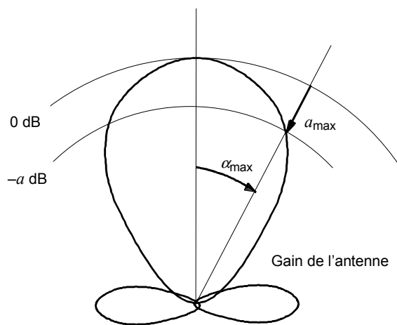
Figure H.2 – Calcul de la réduction de gain résultante a
